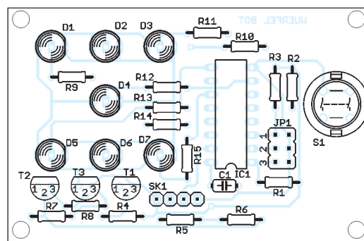
Bild 6: Bestückungsplan der zweiseitig ausgeführten LED-Baugruppe; Abmessungen 68 mm × 44 mm, M 1:1
