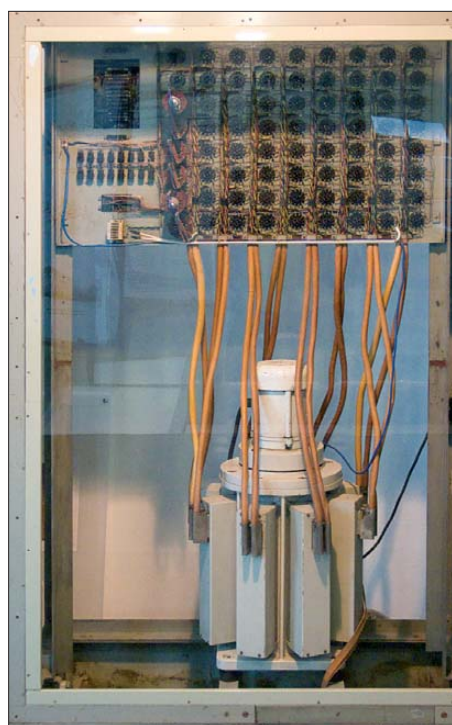
Trommelspeicher des Z22; die Ansteuerung der Schreib-Lese-Köpfe sitzt darüber.
