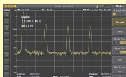
Bild 4: Die Oberwellenunterdrückung beträgt im Originalzustand knapp 20 dB.
