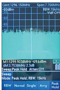
Bild 5: Störnebel am Plastikstecker des HDMI-Kabels A
